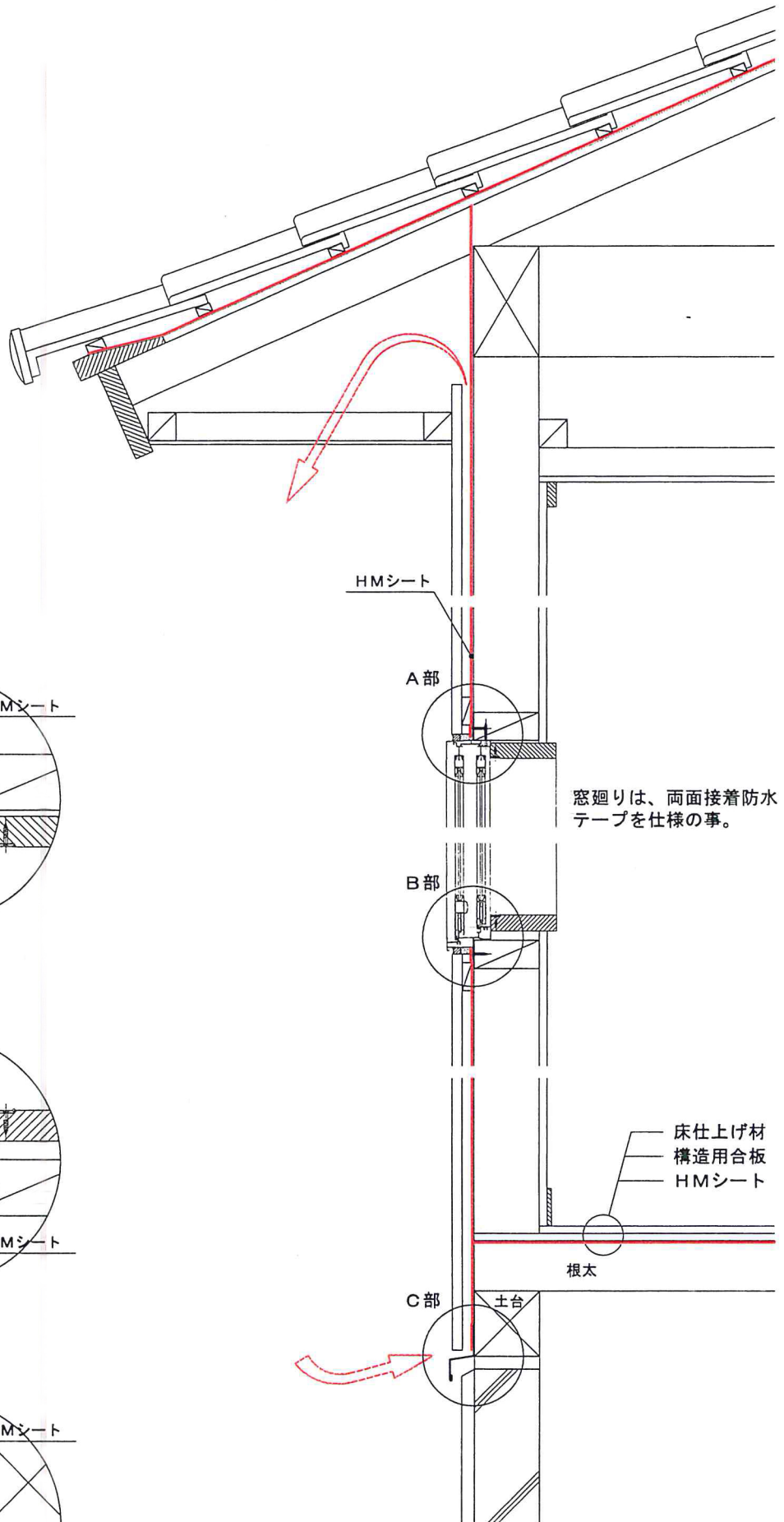
断面施工標準図
