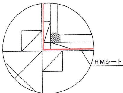
入隅部詳細図
