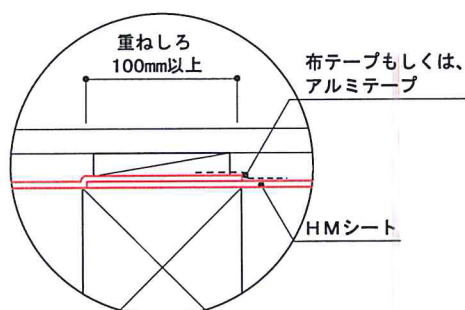
縦ジョイント部詳細図
