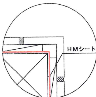
出隅部詳細図
