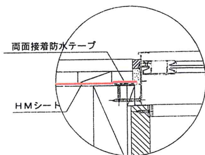
窓廻り部詳細図
